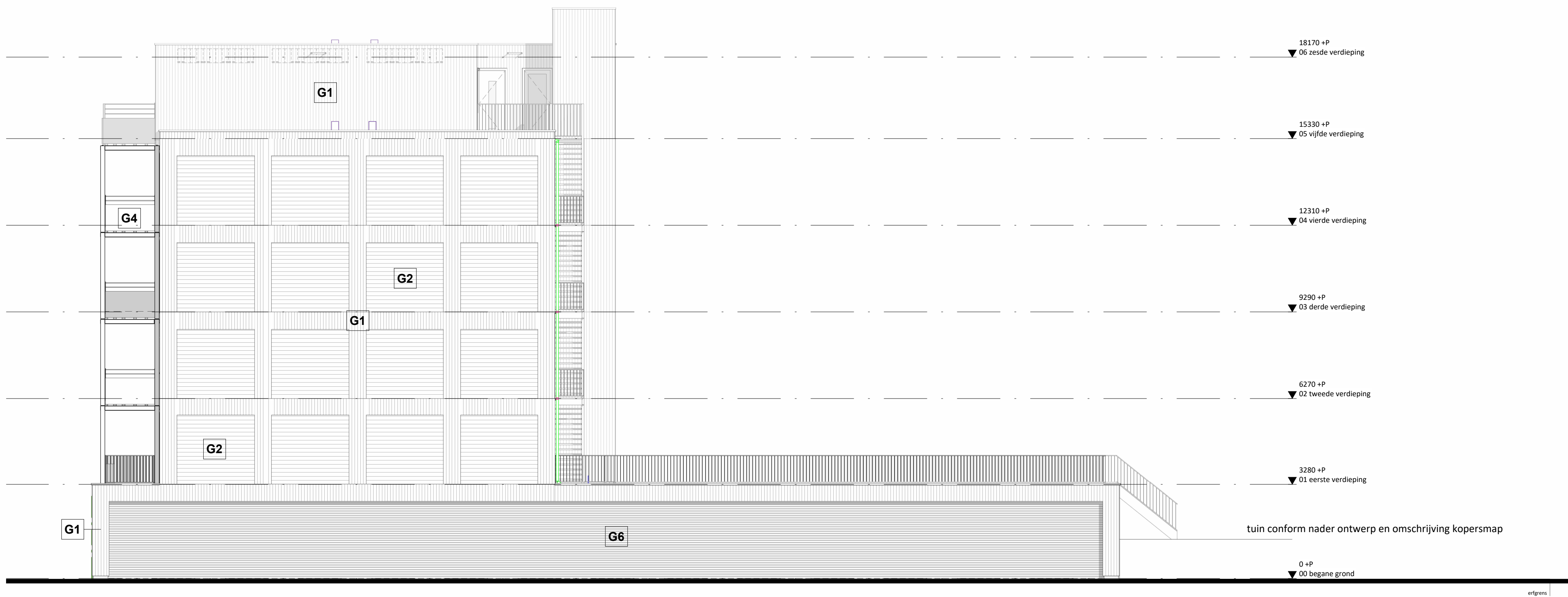
Westgevel
