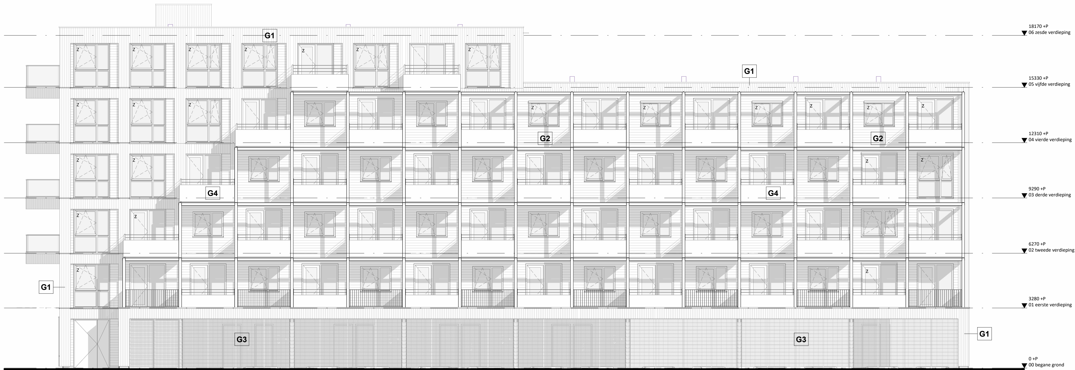
Noordgevel
