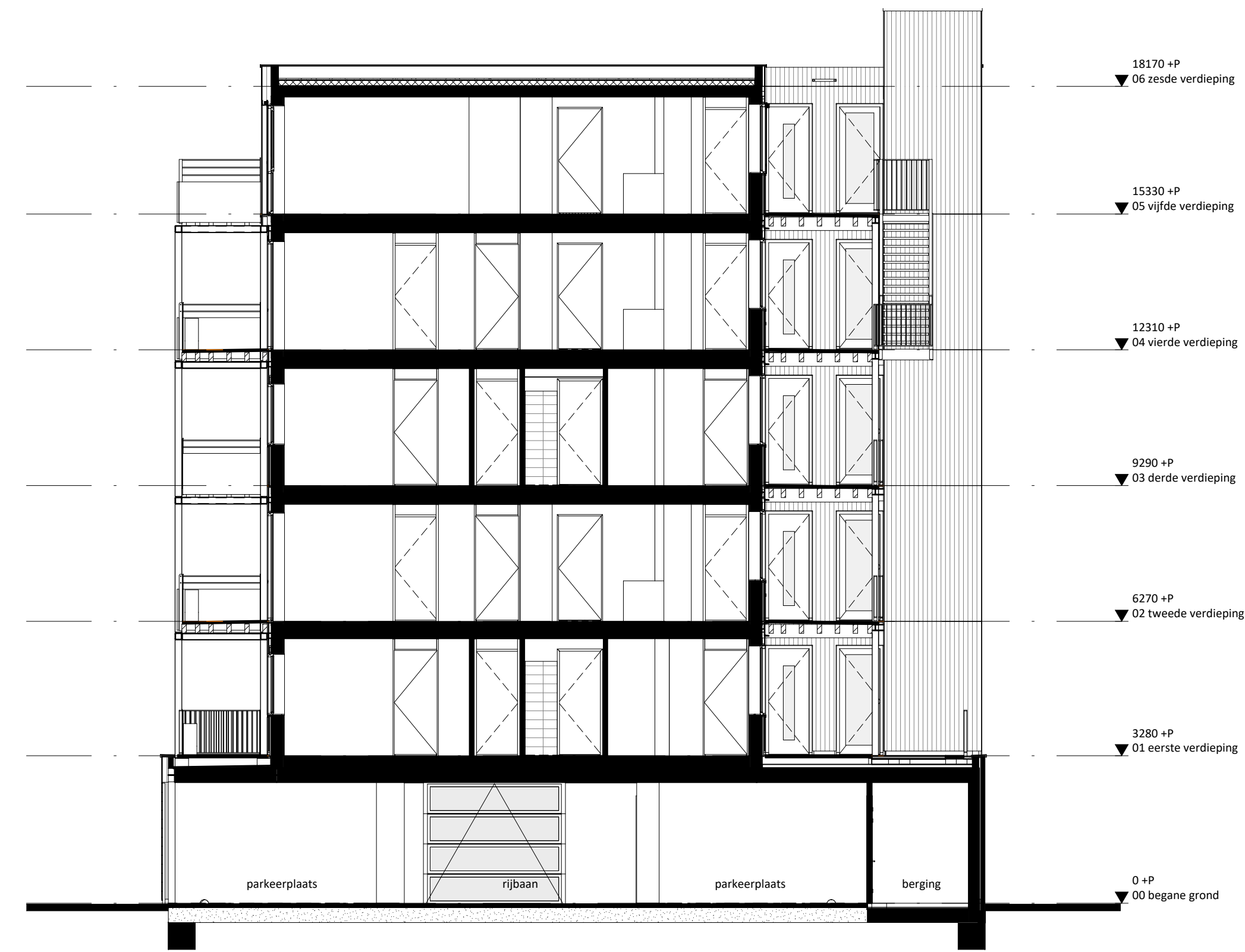
Doorsnede B-B
