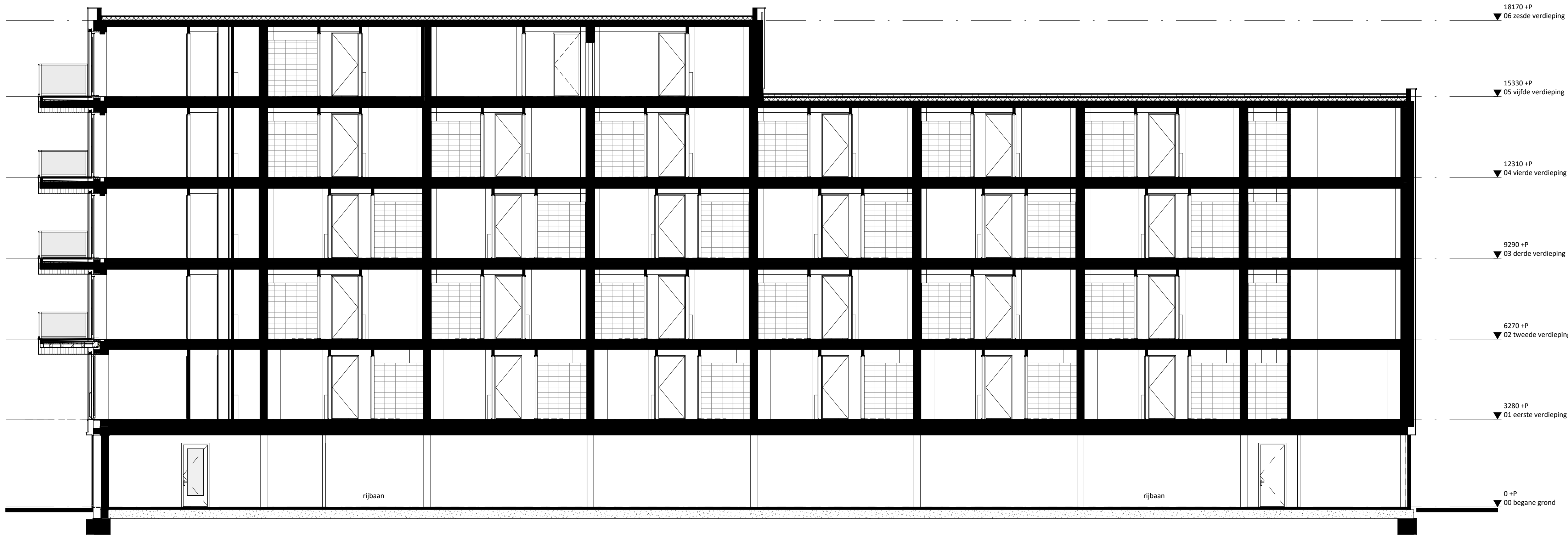
Doorsnede A-A
